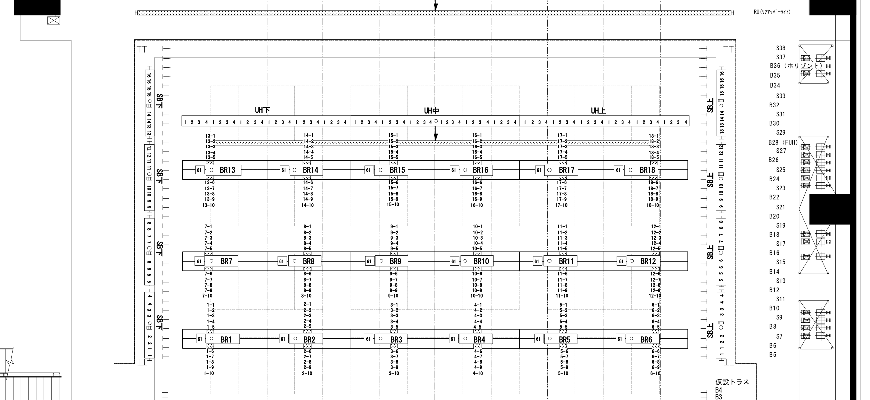
世田谷区立図書館 Overhead 回路図
